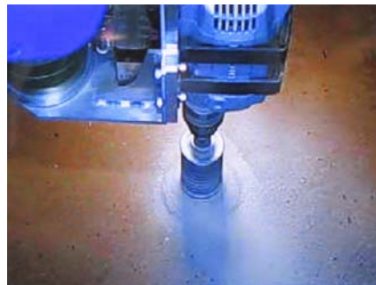
図7 コア切削
