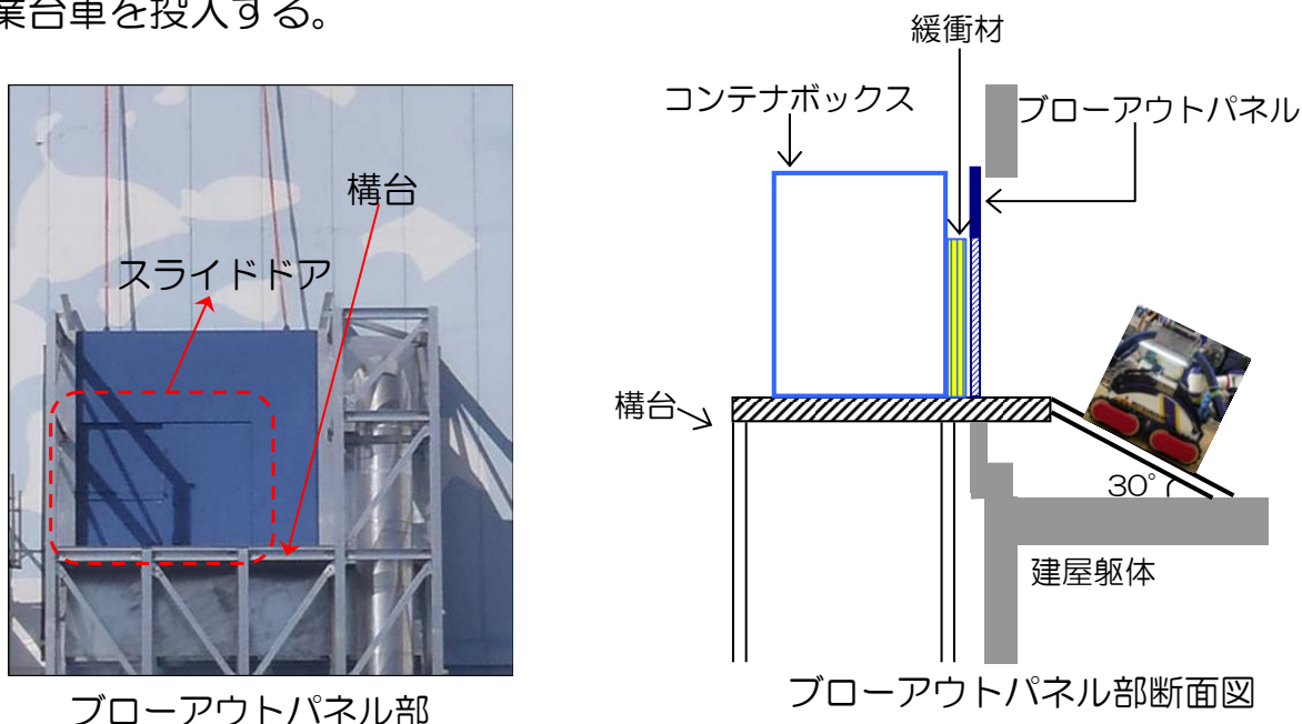
図 ブローアウトパネル部からの調査工法概要
