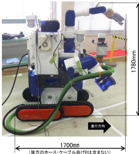
除染ヘッド/ホース取付け時(走行姿勢)の寸法
