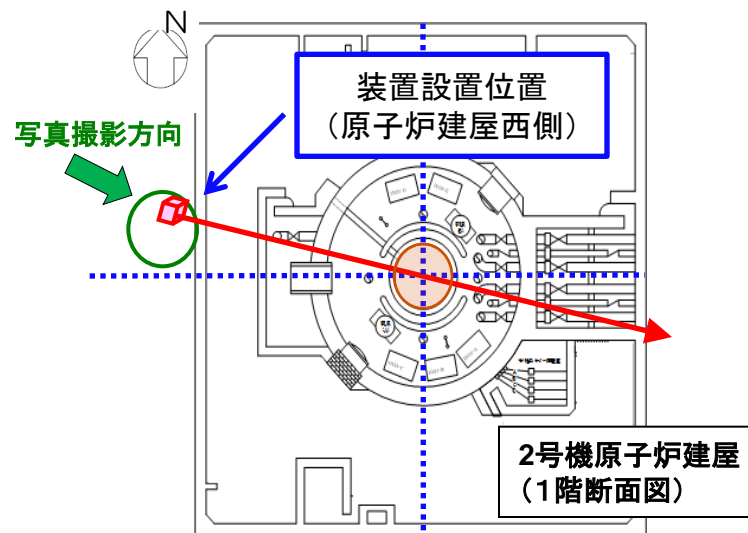
ミュオン測定装置 設置位置
