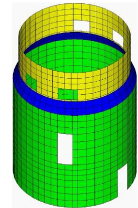
PRVペデスタル 耐震評価モデル
