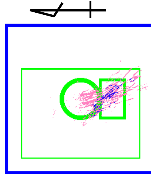
図2 炉心高さ断面 高吸収体の交点無し
