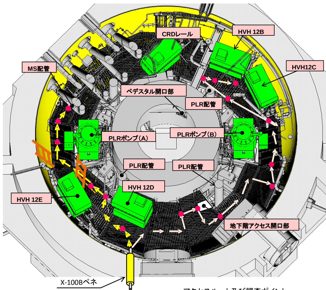
アクセスルート及び調査ポイント
