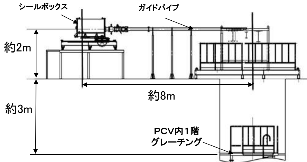
PCV内挿入/回収用模擬体(側面図)
