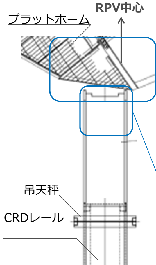
PCV平面図
