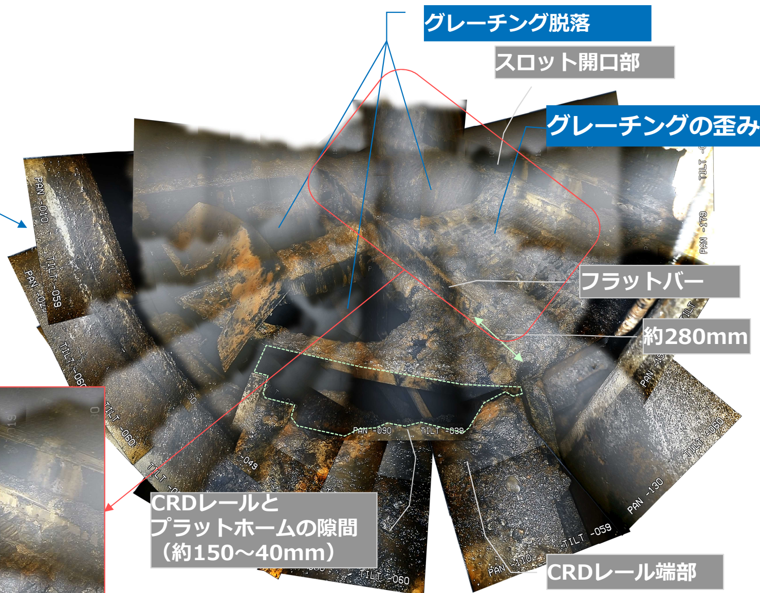
2号機のペデスタル内調査画像
