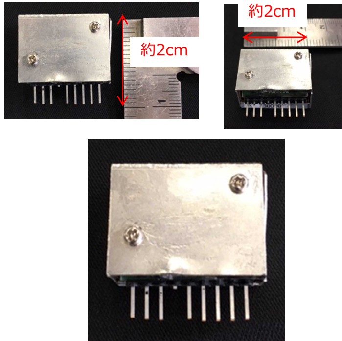
線量計外観
