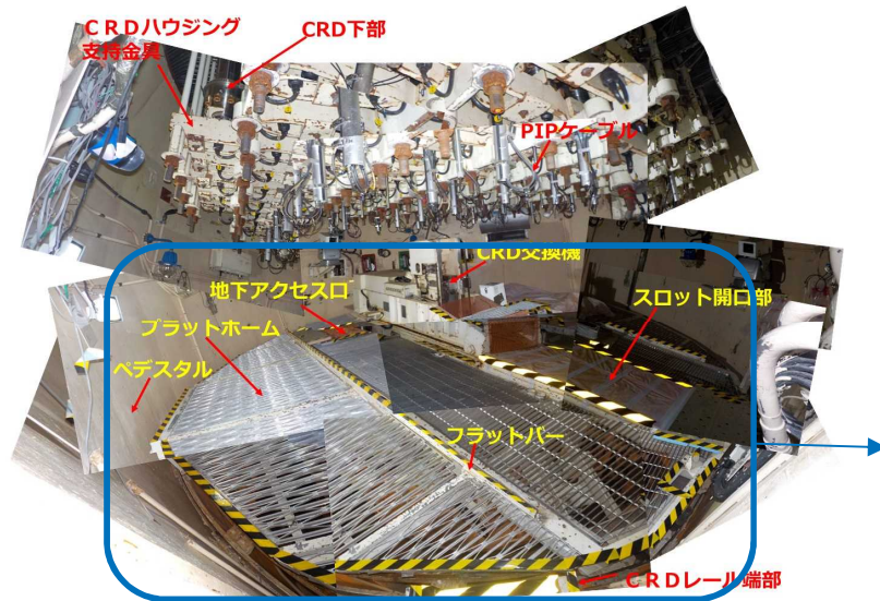
(参考) 5号機のペデスタル内
