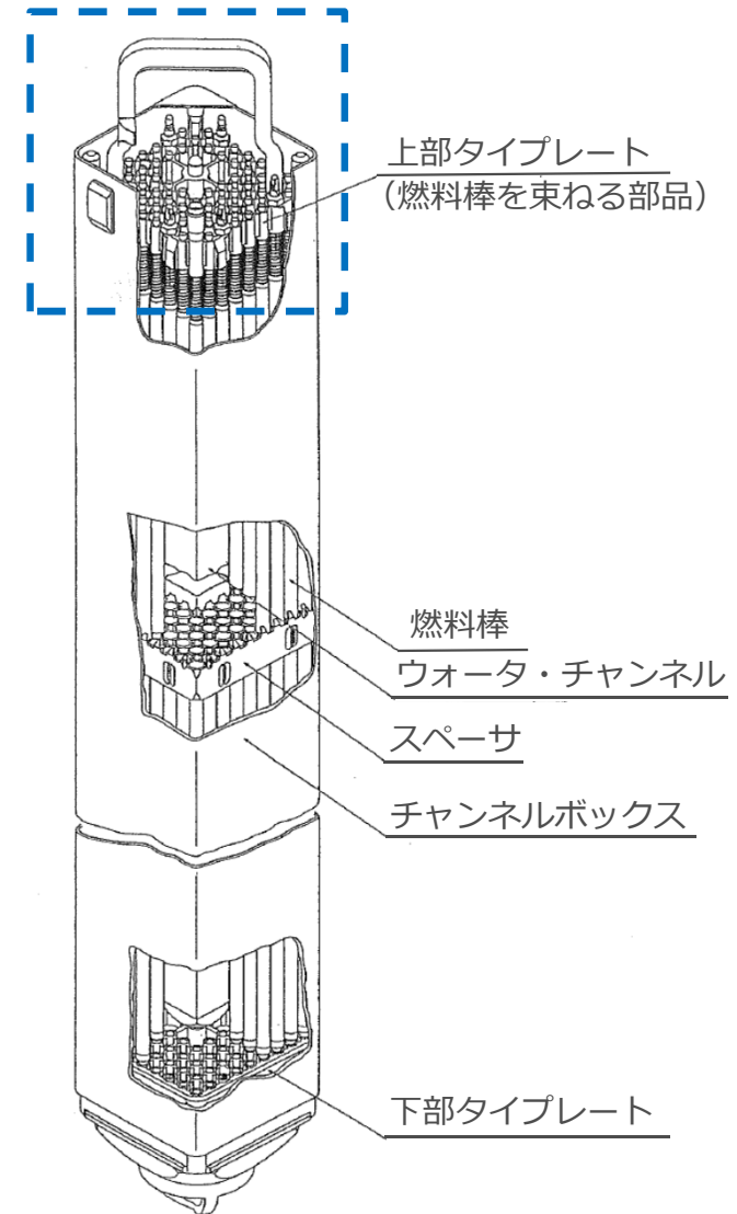
燃料集合体概要図
