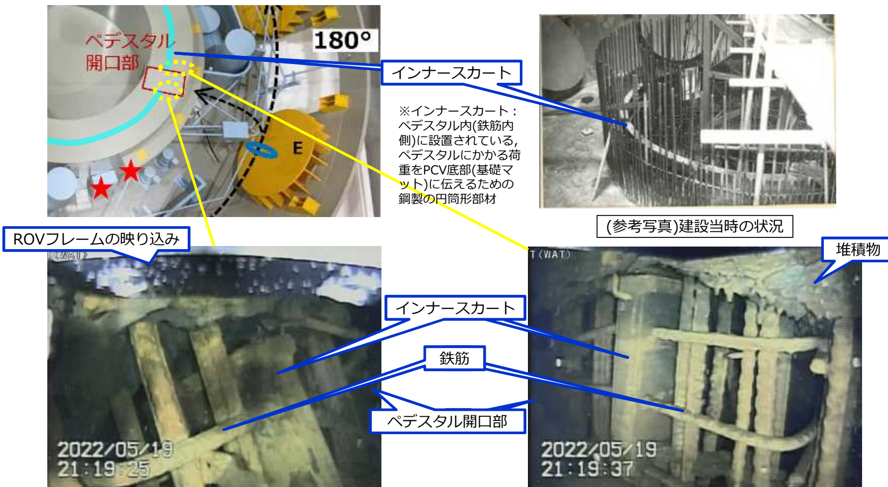
写真1.ペDESTAL開口部(左側基礎部)の状況
